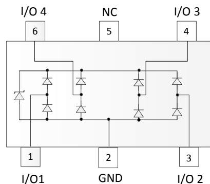
SOT23-6
